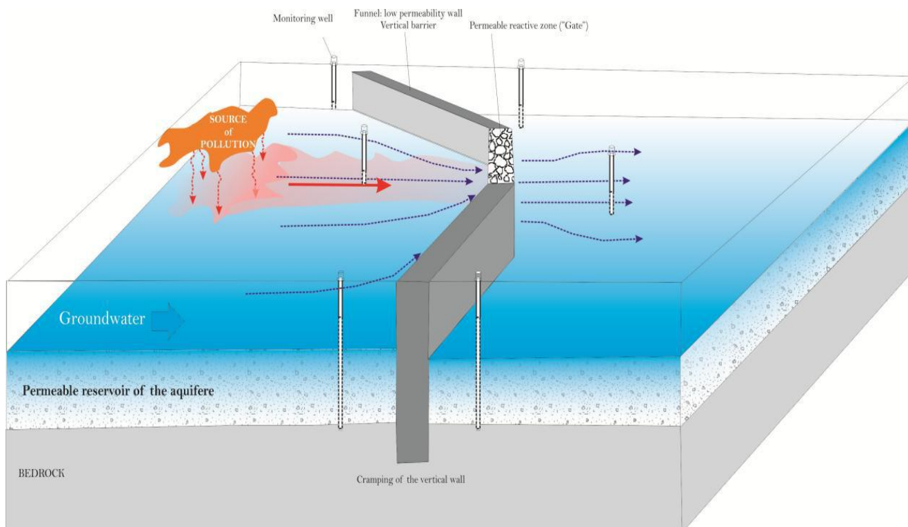
Рис. 14: Принцип ПРБ - "воронка и ворота" (адаптация из работы Colombano et al, 2010)
