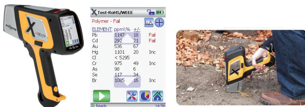
Рис. 2: Портативный рентгеновский флуоресцентный анализатор Olympus Delta с примером показаний для содержания металлов в полимерах на экране. Источник: www.innovx.com
