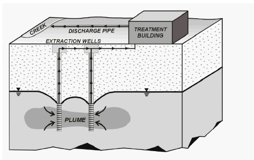
Рис. 13: Принципы откачки и очистки. Факультет геологических наук Техасского сельскохозяйственно-механического университета
